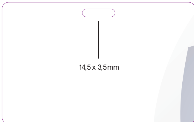
agujero oblongo
